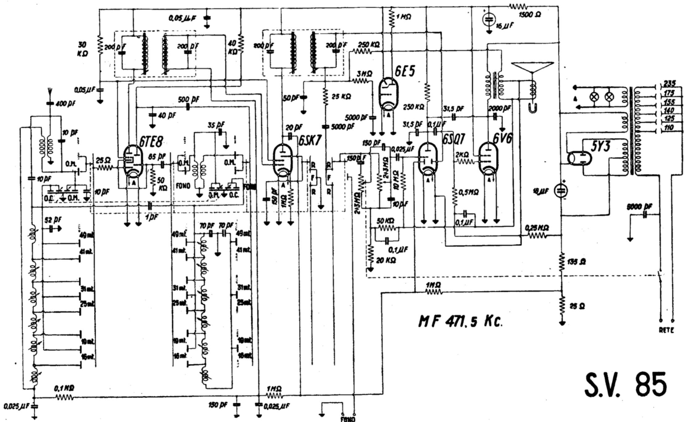
MAGNADYNE RADIO - Mod. SV 85 - Gamma onde medie intera, sei gamme onde corte con bobine in serie. Media frequenza, 471,5 kc/s. Doppia reazione negativa. Sensibilità media 30 microvolt. Potenza d'uscita 4 W. Altoparlante magnetodinamico. Consumo 60 W.
